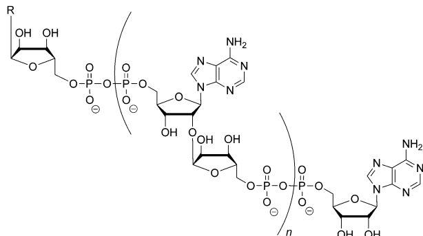
Scheme 1. Structure of linear PAR oligomers.
